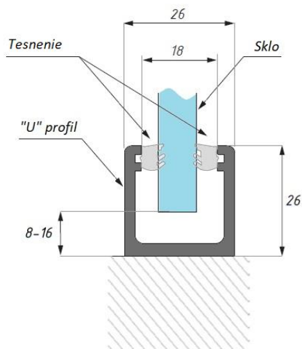
Nerezový „U“ profil a tesnenie
