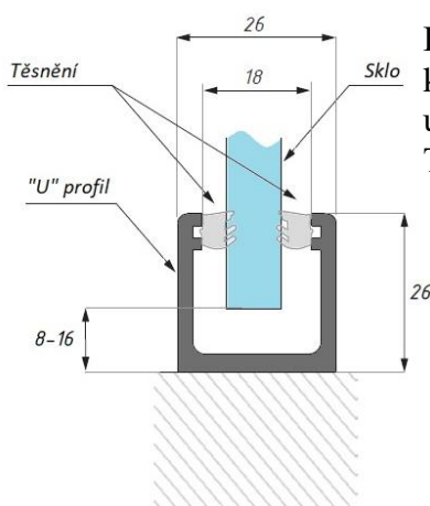
Hliníkový „U“ profil a těsnění
