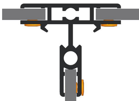
S300 szekrény részlet: Hátsó T profil keresztmetszete
