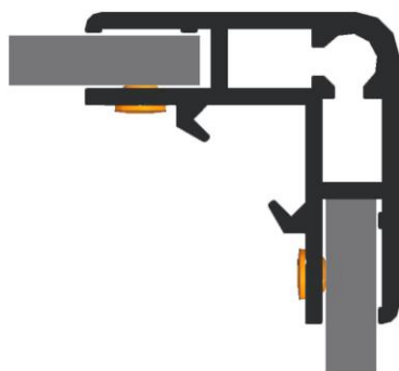
S300 szekrény részlet: Oldalsó alu.profil keresztmetszet
